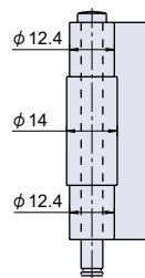
取付参考図
