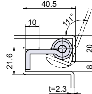
取付参考図
