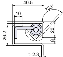
取付参考図
