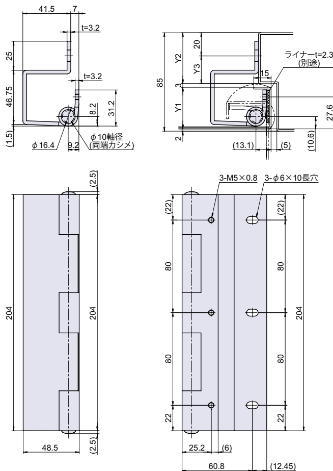
取付参考図
