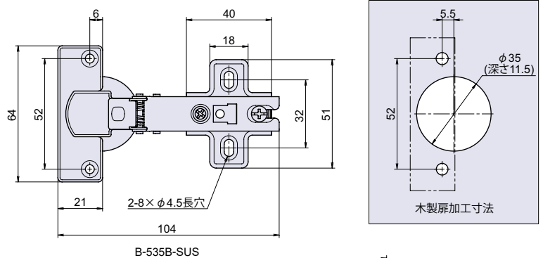
取付参考図
