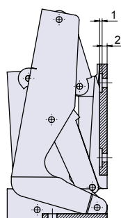
断面図 A-A
