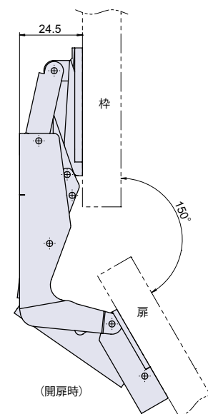
取付参考図
