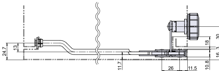
取付参考図 L-251+L-416
