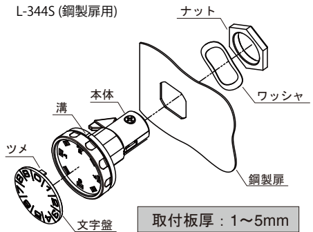
L-344S (鋼製扉用)
