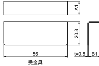
受金具
