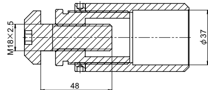
断面図A-A
