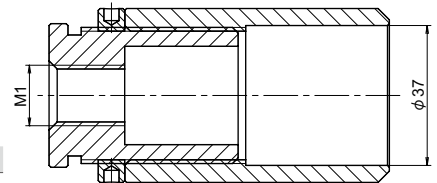
断面図 A-A
