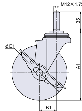
PC-87S ※図面はストッパー付です。
