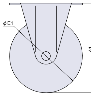
PC-86-N (ナイロン車)
