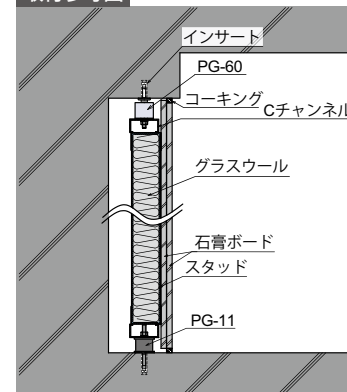
取付参考図
