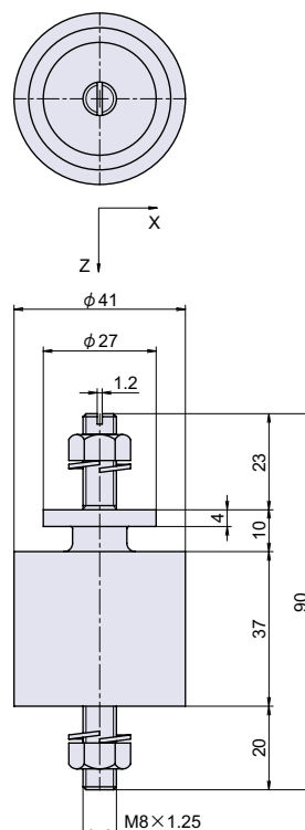
取付参考図
