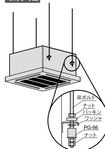
取付参考図
