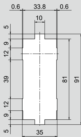
鋼製扉
