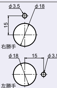
PH-30-3 スタンダード型 ハンドル
