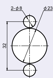
PCH-19-2 PCH-19A-2 防水ハンドル
