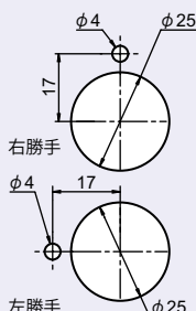
PH-42K PH-42 ブラカンハンドル
