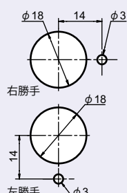
PH-3-2 管型ハンドル
