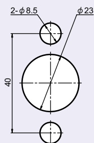
PCH-19-1 防水ハンドル
